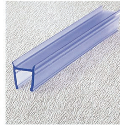
B027 180° 玻璃侧挡水条 配套: 8、10mm 玻璃 8mm a=10 b=5 10mm a=11 b=7
